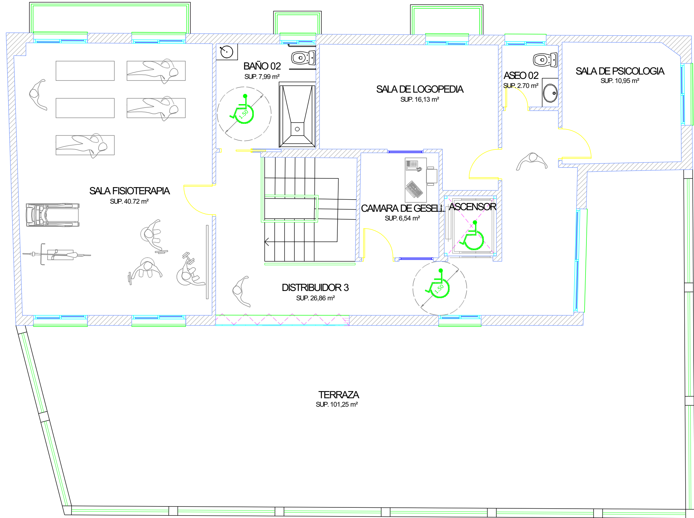
PLANTA ALTA SUP. CONSTRUIDA: 153,11 m 2
